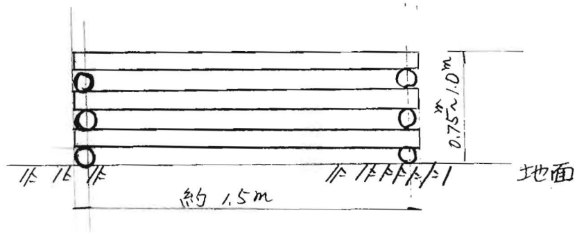
図-2 側面図(Aが見た所)
